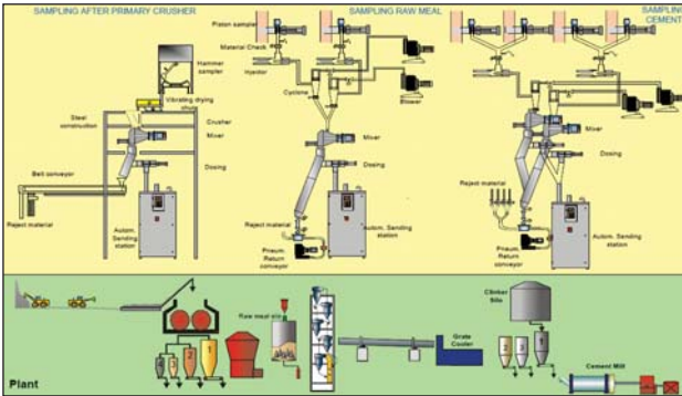
Shema automatskog uzorkovanja
